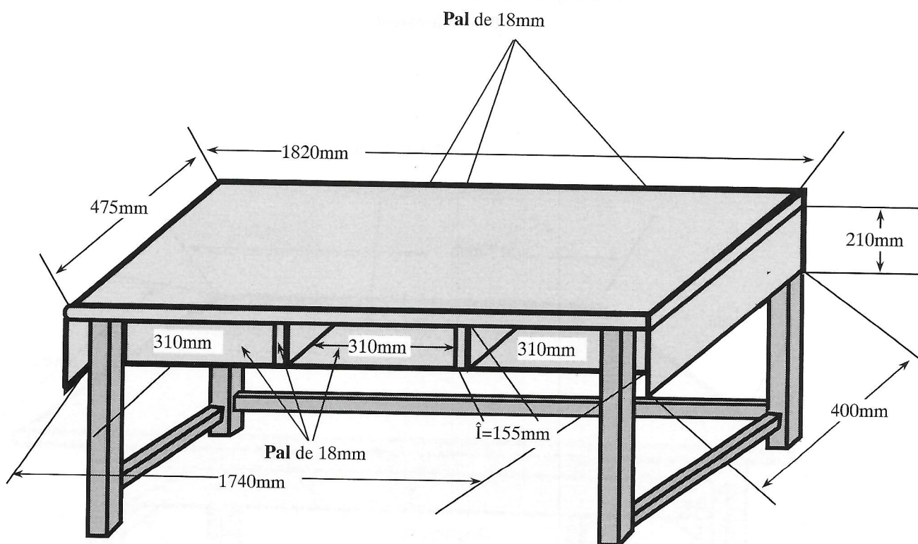
Schița 6 (propus)
