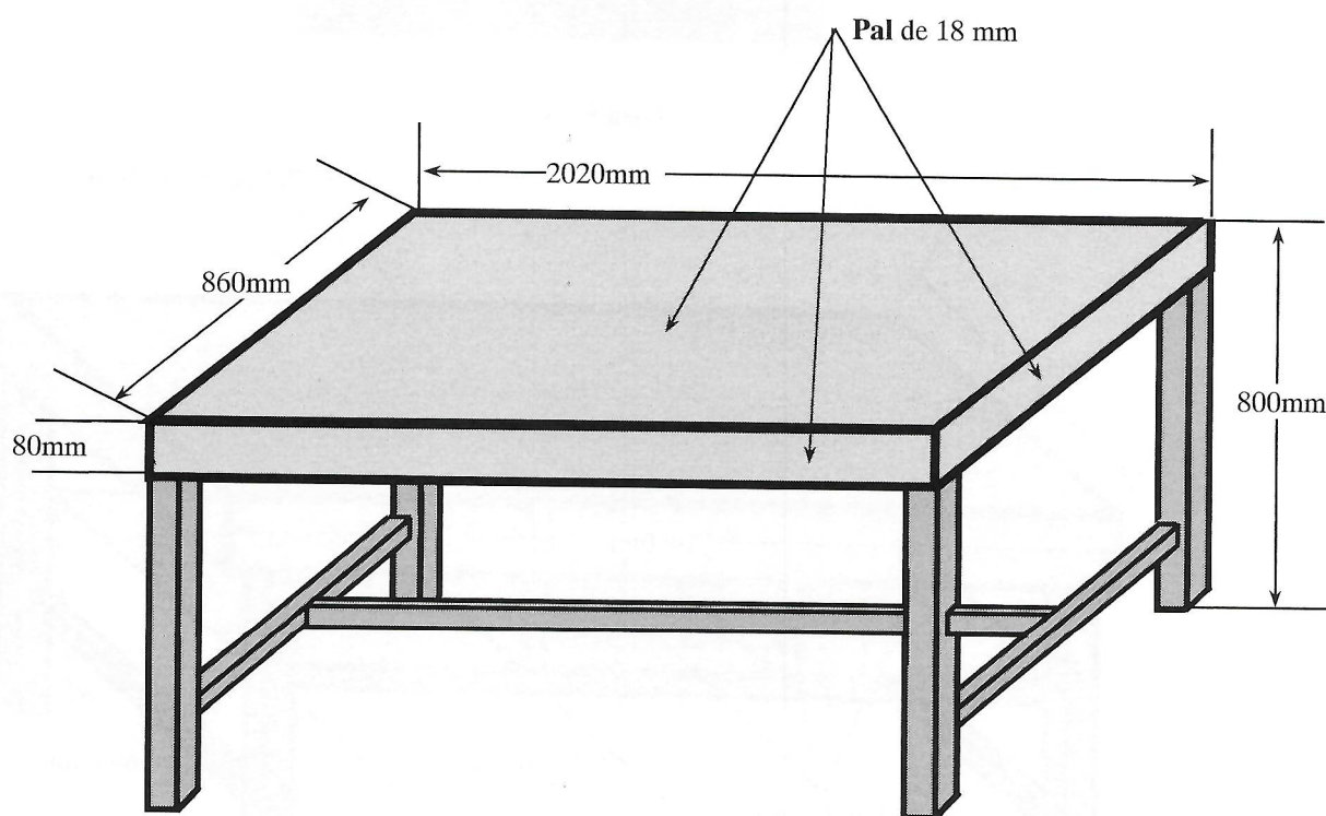
Schița 4 (propus)
