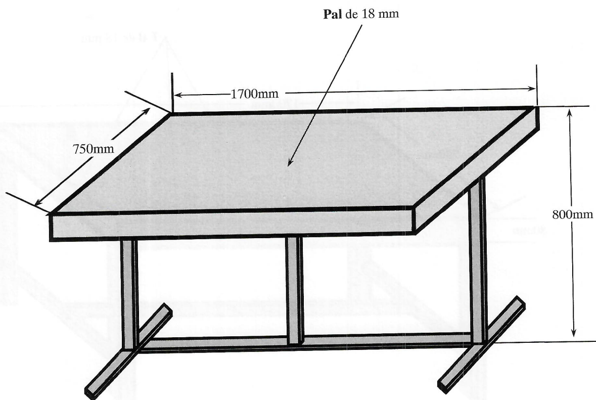
Schita 9 (propus)
